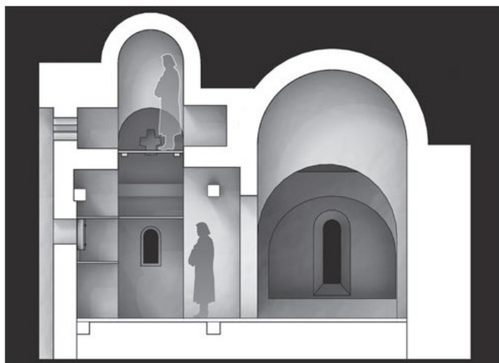
Илл. 10. Северный компартимент хор Спасской церкви Евфросиньева монастыря в Полоцке Деревянные конструкции XII в. Продольный разрез с видом на юг Реконструкция П. Зыкова
